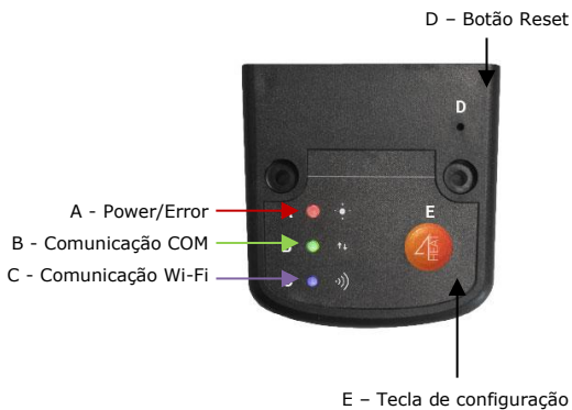
Figura 6 – Módulo Wi-Fi
