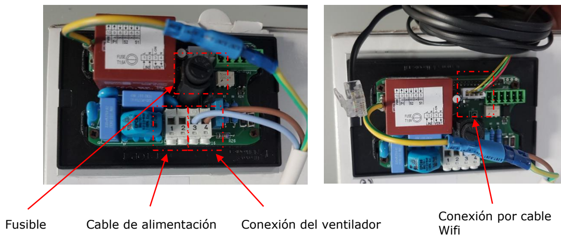
Figura 56 – Diagrama de conexión de componentes
