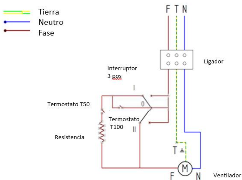
Figura 41 – Esquema eléctrico
