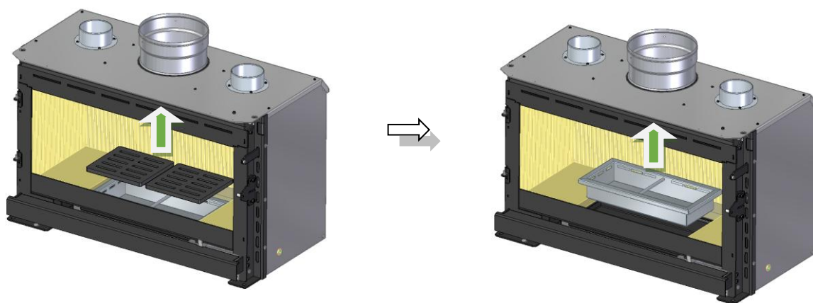
Figura 32 – Desmontaje del cajón de las cenizas
