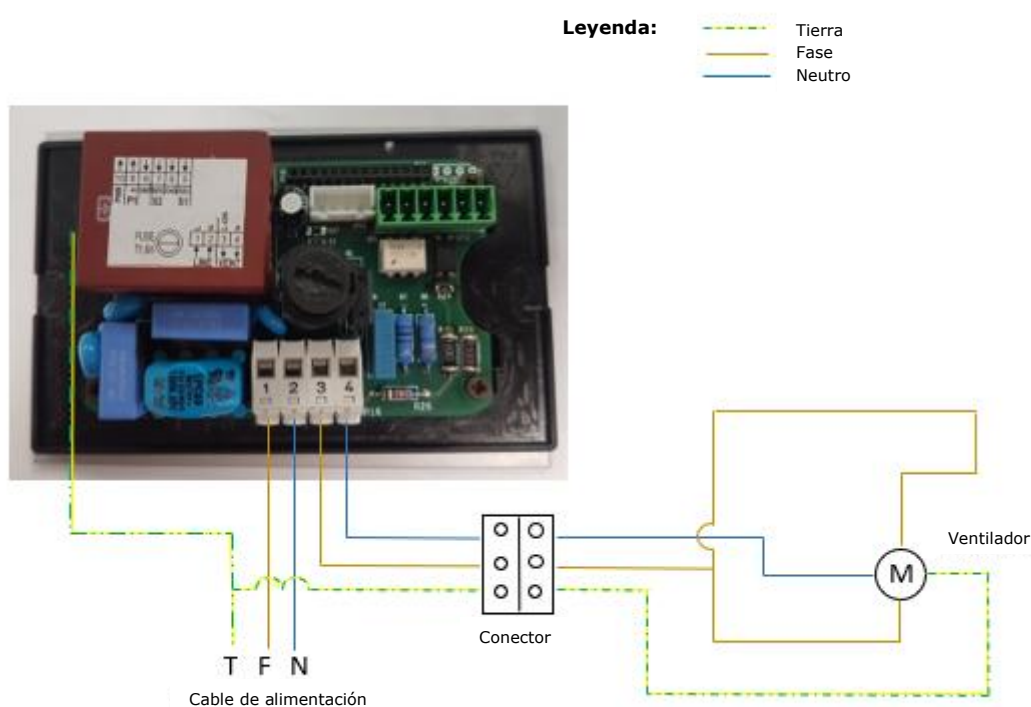
Figura 54 – Esquema eléctrico de la ventilación tangencial
