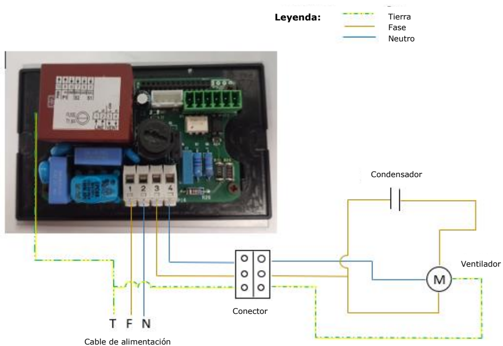
Figura 55 – Esquema eléctrico de un ventilador centrífugo
