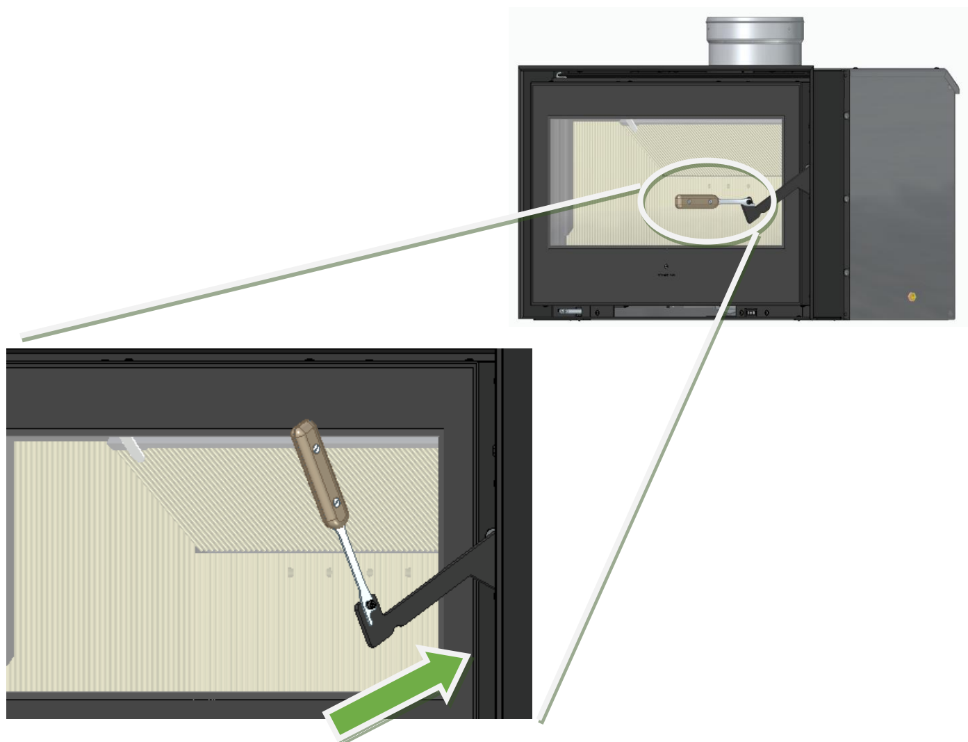
Figure 26 – Fermeture de la porte
