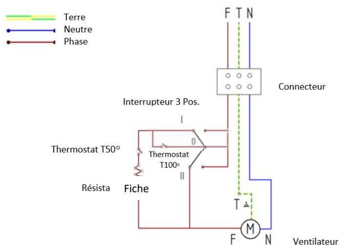
Figure 41 – Schéma électrique
