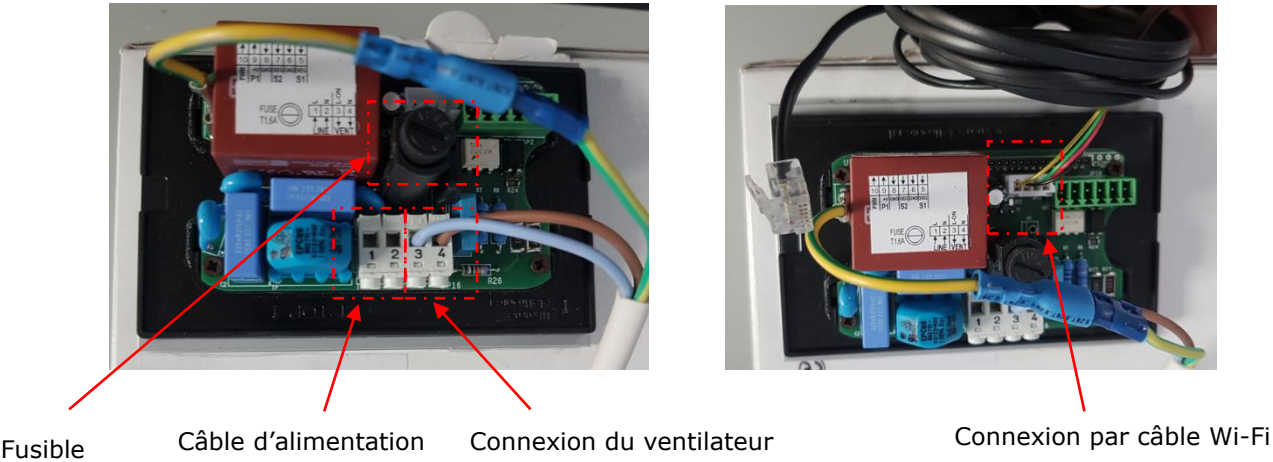
Figure 56 - Schéma de connexion des composants
