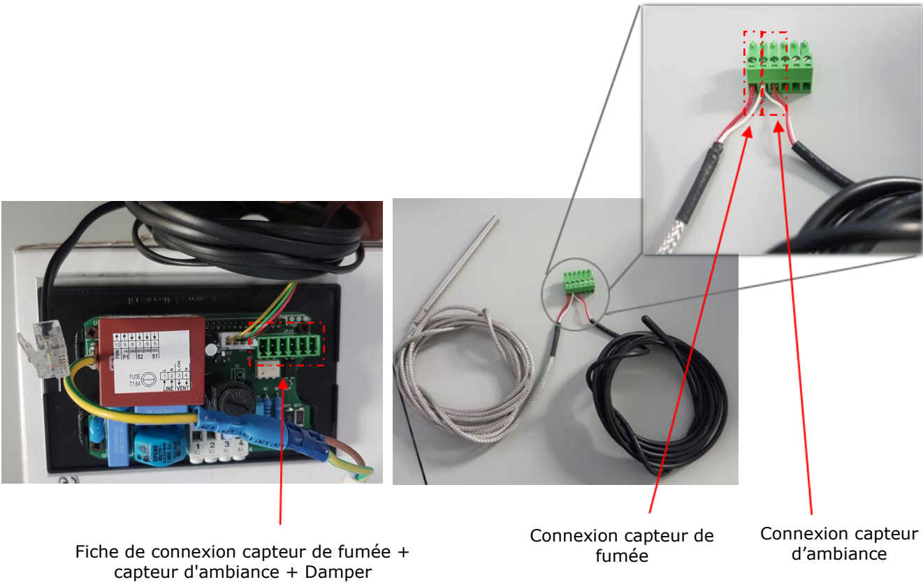
Figure 57 - Schéma de connexion des composants
