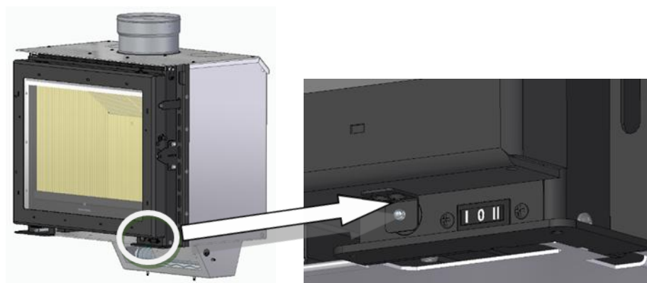
Figure 53 – Réglage de la poignée de porte, fonctionnement par micro-interrupteur
